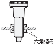
分度销 GN 613
